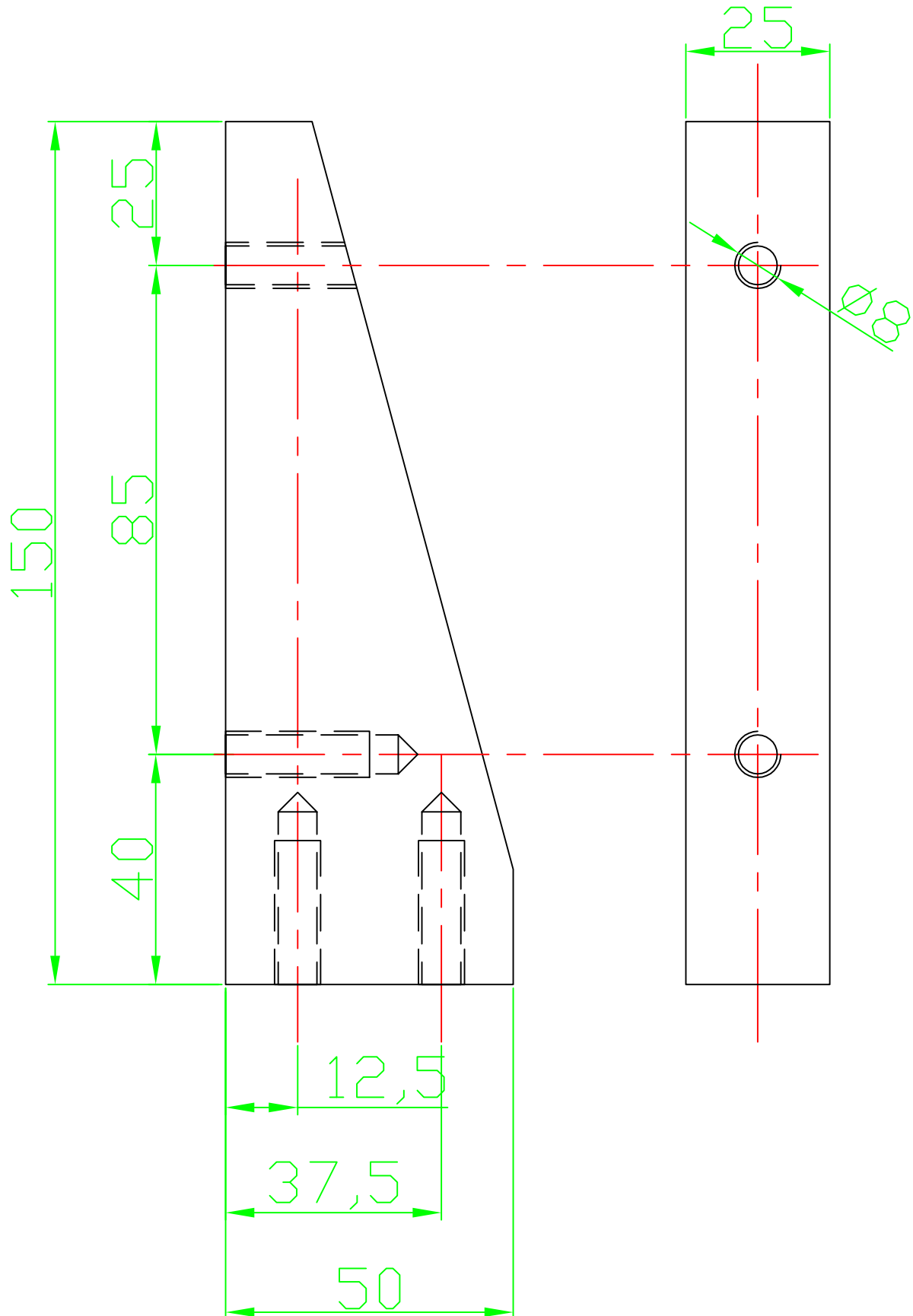
Gousset support Axe Y
